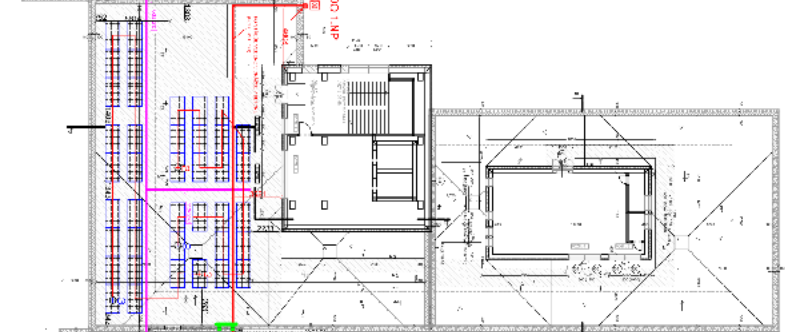
DETAIL KOLEKTIVNÍHO PŘÍKLEMU
